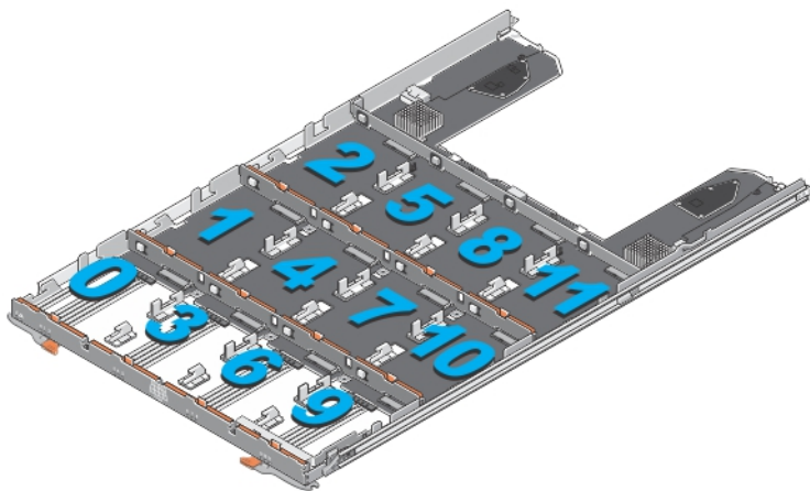
図 14. ディスクドロワーのスロット番号
