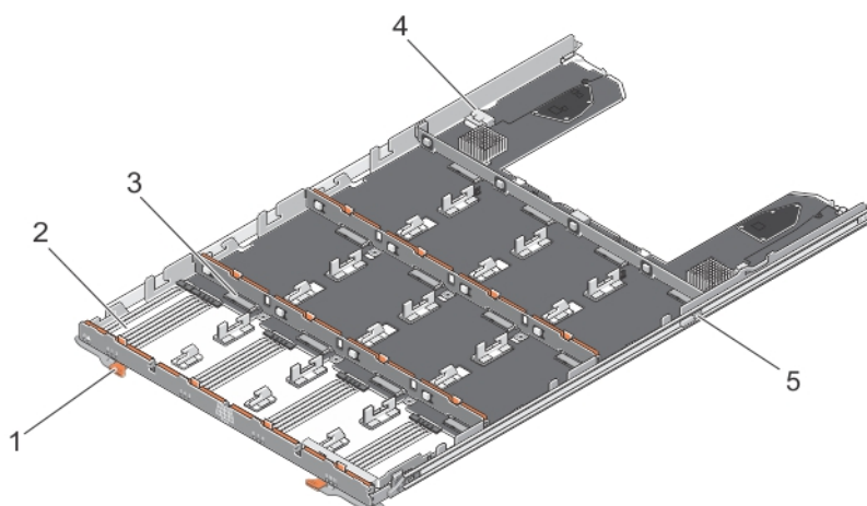
図 11. 物理ディスクドロワーの内部
