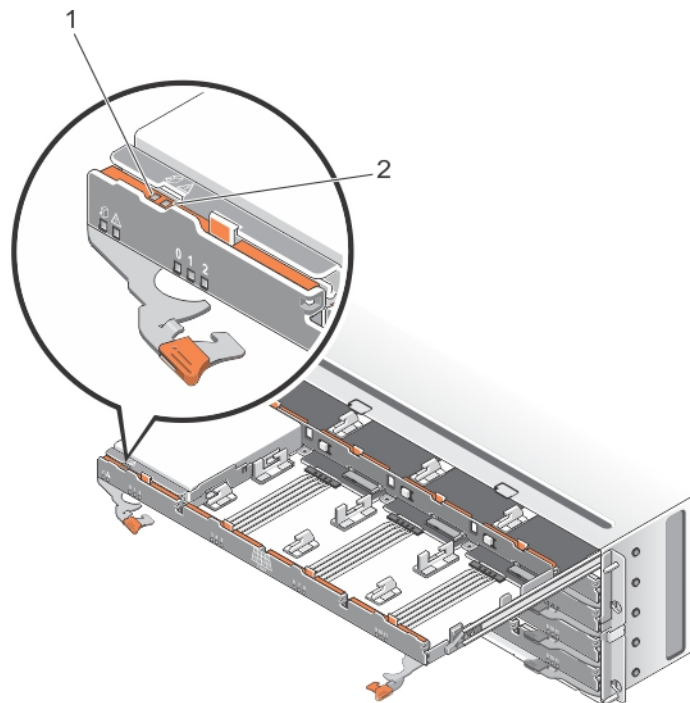
図 7. 物理ディスク LED インジケータ
